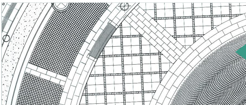
Благоустройство Разбивочный чертеж. План мощения. Баланс площадей.
